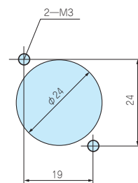
●コネクタ取付穴寸法図
