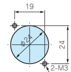
ノートリックコネクタ用 取付穴
